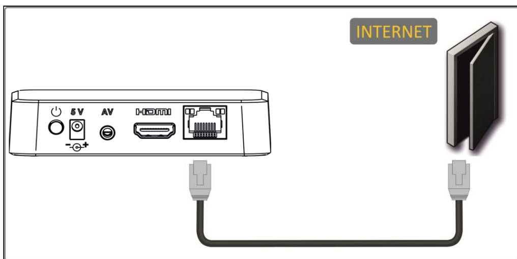
Рисунок 9 – Подключение к сети провайдера без домашнего маршрутизатора
